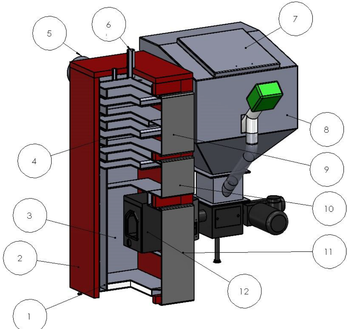
Rys.1. Kocioł "Technix-Pel"
